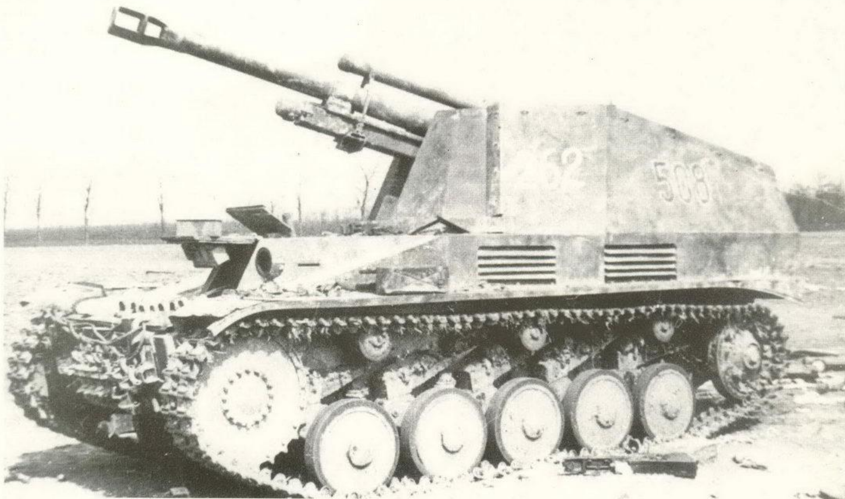
Zdobyte nieuszkodzone działo samobieżne 10,5 cm leFH 18/2 Sf auf Fgst PzKpfw II Sd Kfz 124 „Wespe” z 73. Pulku Artylerii Pancerniej, 1. Dywizji Pancerniej, Węgry, 1945 rok. A captured intact 10.5 cm leFH 18/2 Sf auf Fgst PzKpfw II Sd Kfz 124 „Wespe” SP gun of the 73rd Panzer Artillery Regiment, 1st Panzer Division, Hungary, 1945. [AFOT]
