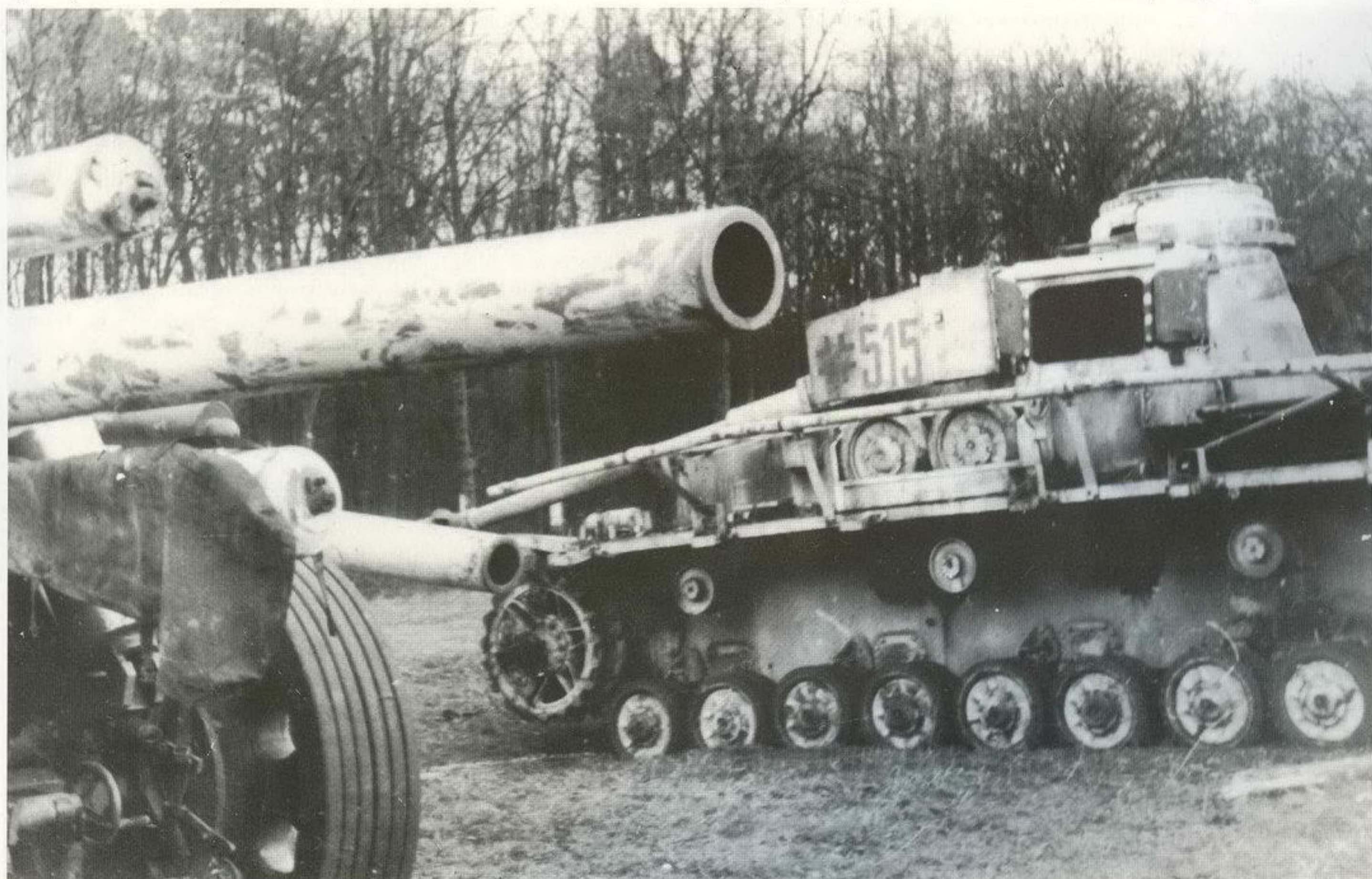
Czołg PzKpfw IV Ausf. J z nr „515” 31. Pułku Pancernego 5. Dywizji Pancerniej, Prusy Wschodnie, marzec 1945 rok. A PzKpfw IV Ausf. J tank coded “515” from the 31st Panzer Regiment 5th Panzer Division, East Prussia, March 1945. [ASKM]
