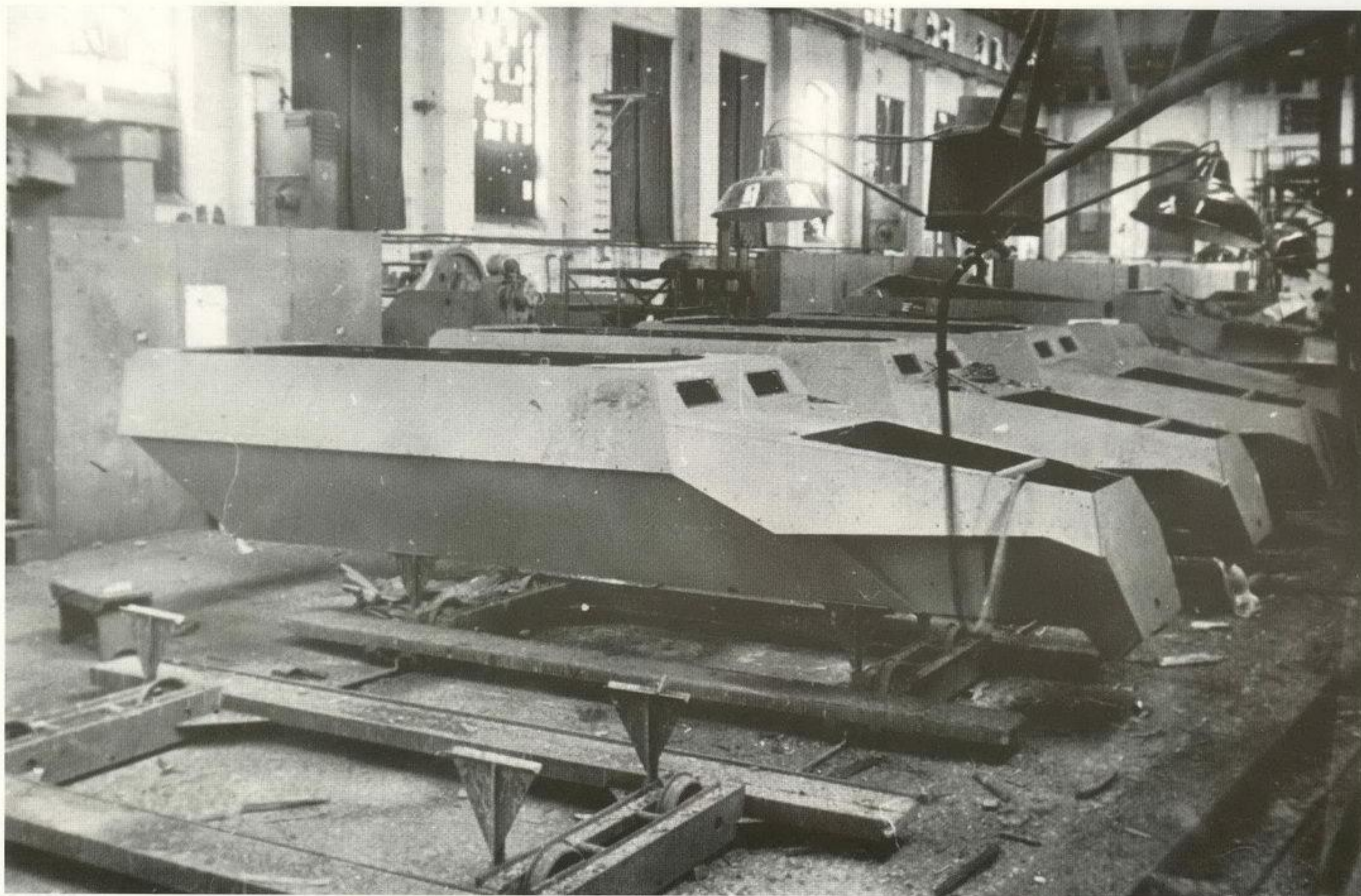
Zdobyte produkowane transportery Sd Kfz 251 Ausf. D w zakładach Schihau w Elblągu w lutym 1945 roku. The captured assembled Sd Kfz 251 Ausf. Ds APC seen in Schihau plant in Elbing (now Elbląg in Poland), East Prussia, February 1945. [ASKM]
