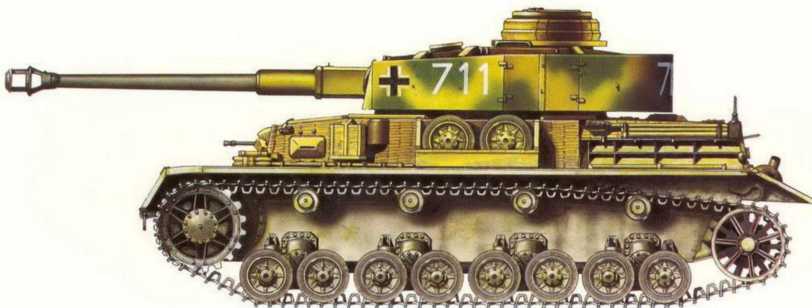
PzKpfw IV Sd Kfz 161/2 Ausf. J z 35. Pułku Pancernego, 4. Dywizji Pancerniej, Gdańsk, marzec 1945 roku. PzKpfw IV Sd Kfz 161/1 Ausf. H tank from the 35th Panzer Regiment 4th Panzer Division, Danzig, March 1945.
