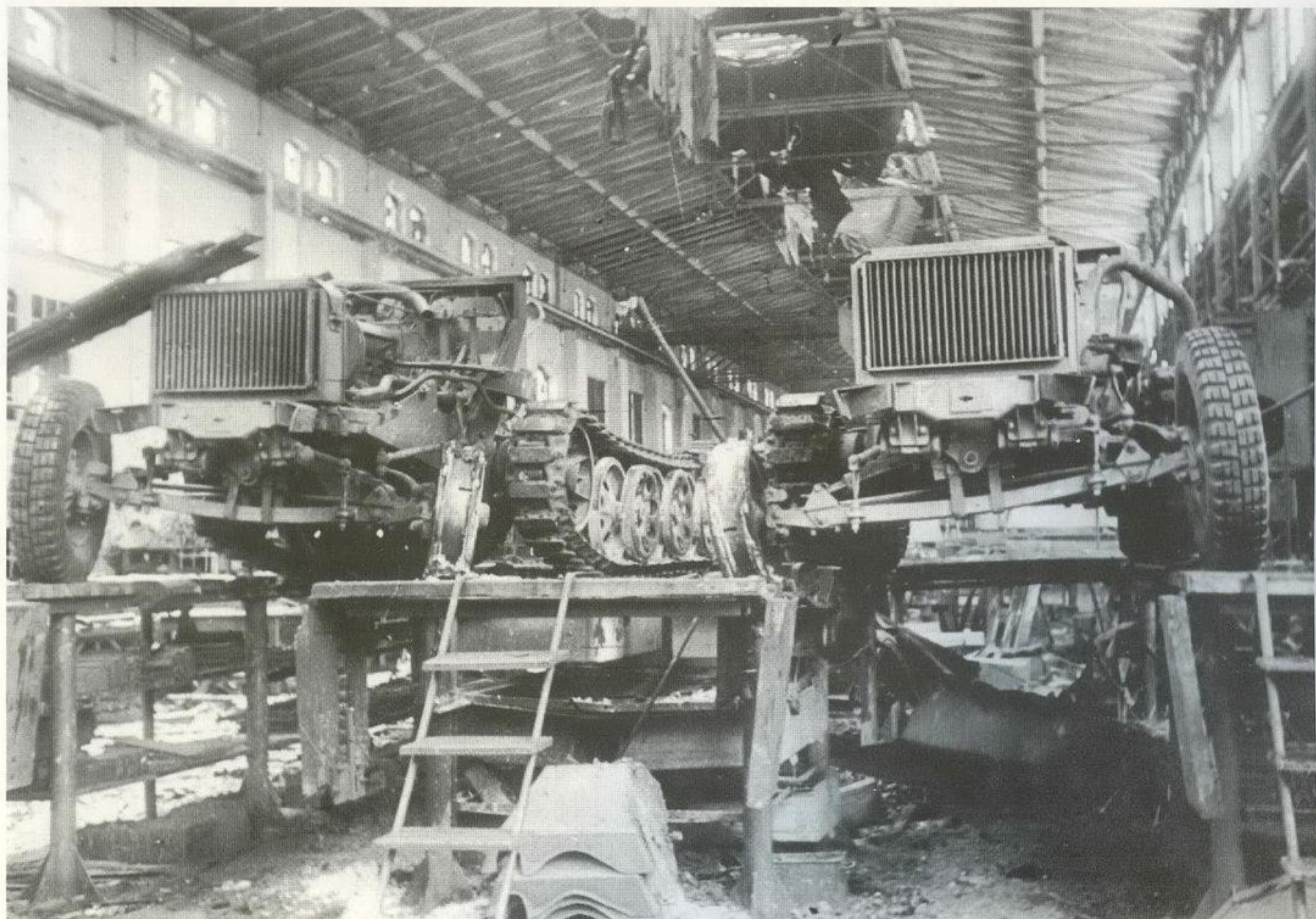
Remontowane podwozia transporterów Sd Kfz 251 w zakładach naprawczych Schihau w Elblągu w lutym 1945 roku. The chassis of the repaired Sd Kfz 251s APC seen in Schihau repair plant in Elbing (now Elbląg in Poland), East Prussia, February 1945. [ASKM]
